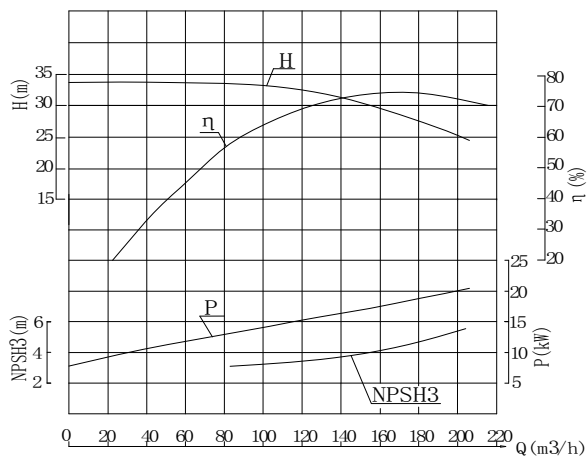
150MD30 型矿用耐磨多级离心泵性能曲线表 (n=1480r/min)
