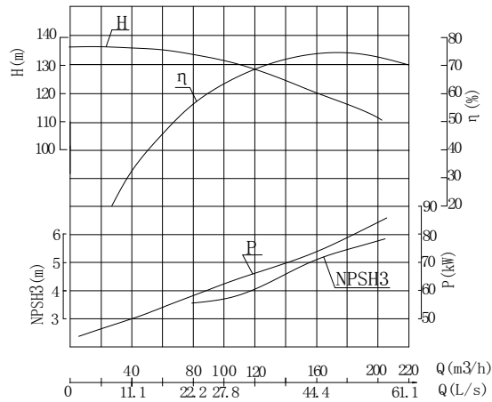
MD160-120 型煤矿用耐磨多级离心泵性能曲线表 (n=2980r/min)
