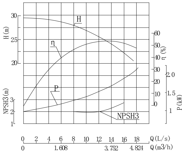
MD12-25 型煤矿用耐磨多级离心泵性能曲线表 (n=2950r/min)
