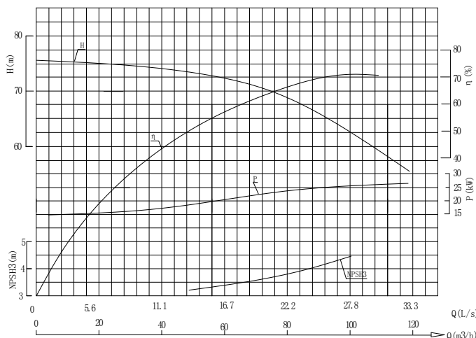
MD85-67 型煤矿用耐磨多级离心泵性能曲线表 (n=2950r/min)
