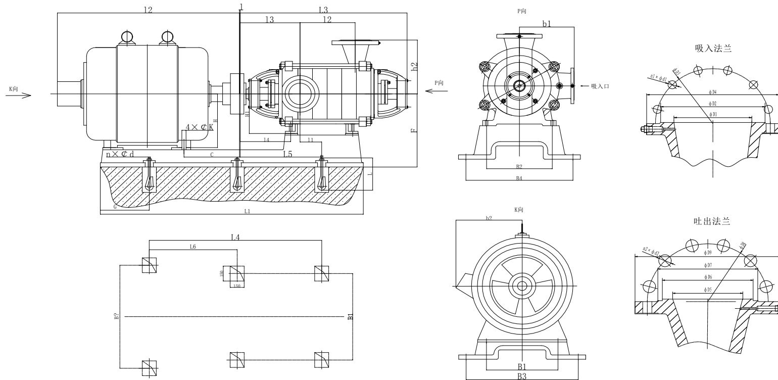
图3 | MD 型矿用耐磨多级离心泵（整体底座）
