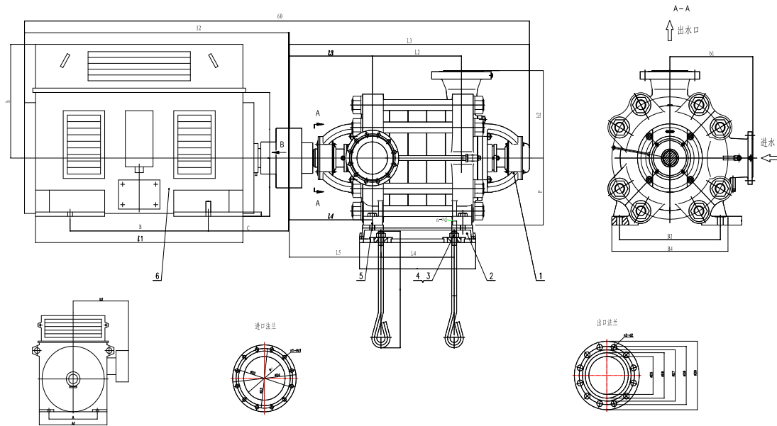
图5 MD型矿用耐磨多级离心泵（独立底座）
