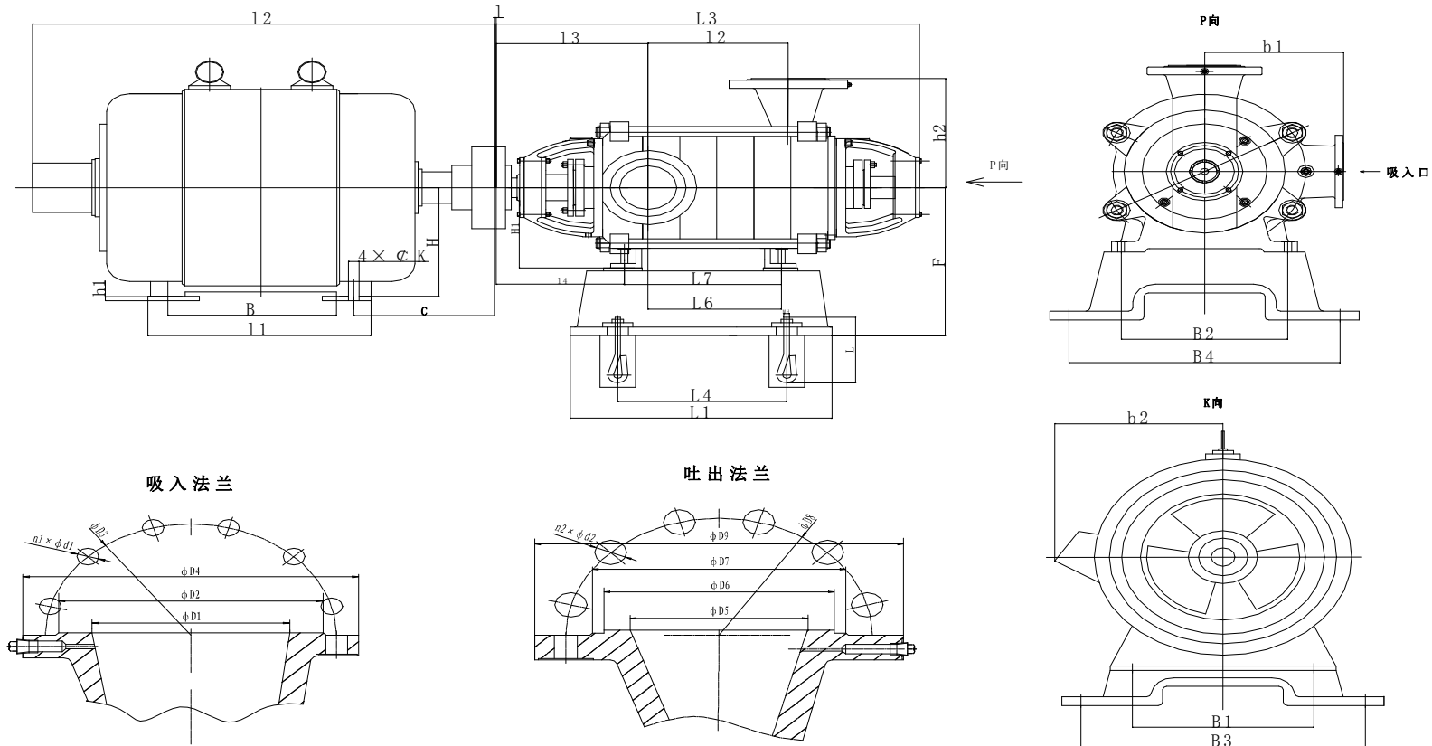
图 4 MD 型煤矿用耐磨多级离心泵（单独底座）
